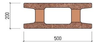
N - tvarovka (normál - priebežná)
