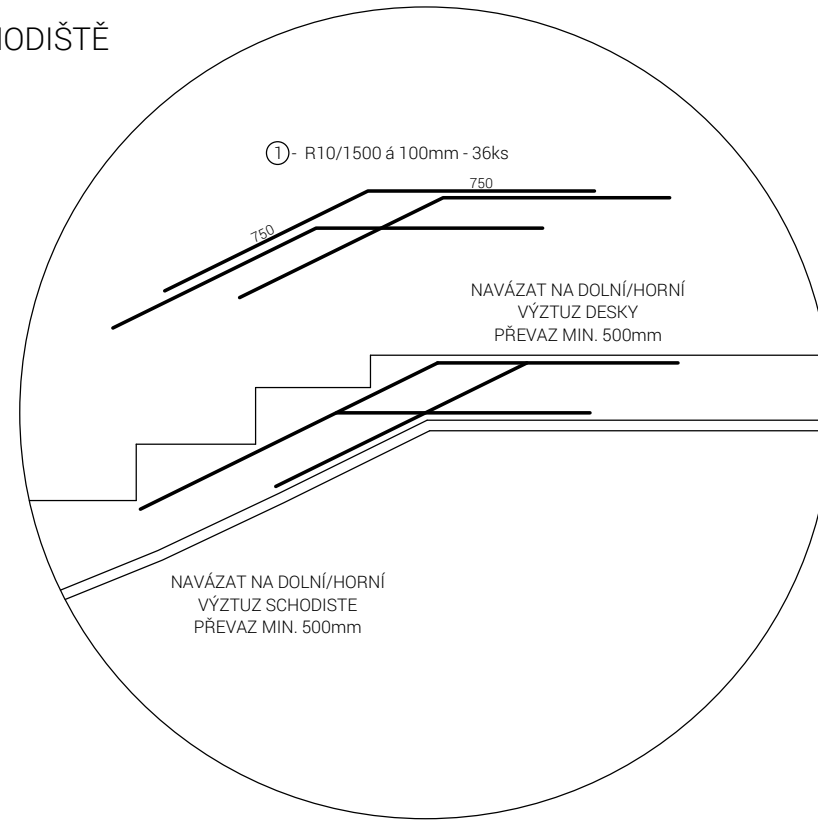
PŮDORYS ARMATURY
